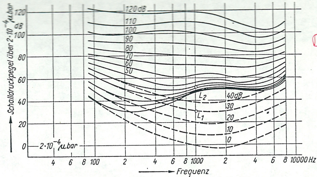
Bild 43a. Schwelennahe Störung der Lautheitsempfindung (positives Recruitment)
