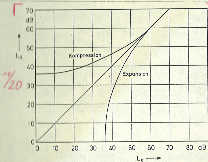
Expansionskurve des Gehörs für einen durch 40 \text{ dB} / \Delta f_g Schmalbandrauschen gedrosselten 1 kHz-Ton (nach ZWICKER 1963)
