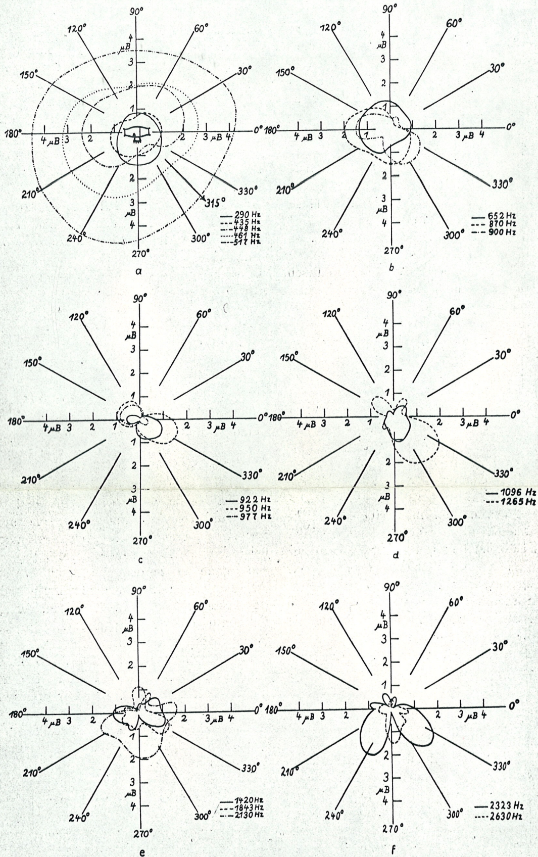
Abb. 16. Richtwirkungsdiagramme der Geige M VII für verschiedene Frequenzen
