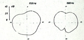
Abb. 6 Polardiagramme zweier Geigen bei 1500 Hz (Stegebene)
