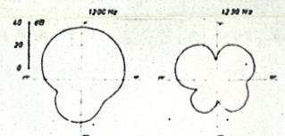
Abb. 7 Polardiagramme zweier Geigen bei etwa 1200 Hz (Stegebene)
