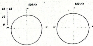
Abb. 4 Polardiagramme zweier Geigen bei 500 Hz (Stegebene)
