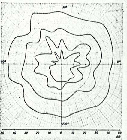
Abb. 10 Polardiagramme des Klanges c''' in der waagerechten Ebene, Flügeldeckel offen, Reflektor unter dem Flügel. Oktavfiltermitte der Kurven von außen nach innen: 1000 Hz 2000 Hz 4000 Hz 4000-8000 Hz 8000 Hz
