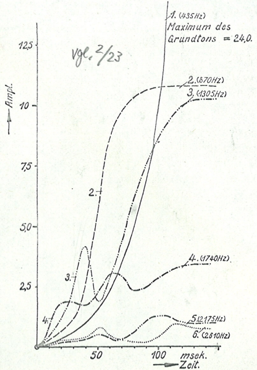
Abb. 25. Entwicklung der Teiltöne der Geige a_1 , 435 Hertz
