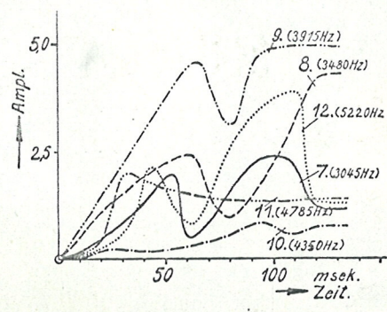
Abb. 25. Entwicklung der Teiltöne der Geige a_1 , 435 Hertz
