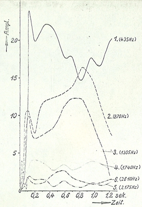
Abb. 26. Änderung der Teiltonamplitude während des Geigenklanges
