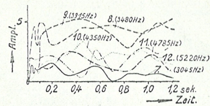
Abb. 26. Änderung der Teiltonamplitude während des Geigenklanges
