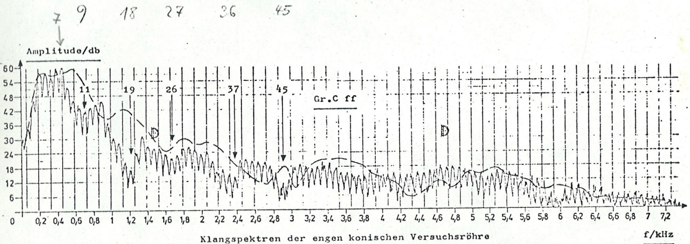
Klangspektren der engen konischen Versuchsröhre (Dulzianrohr)
