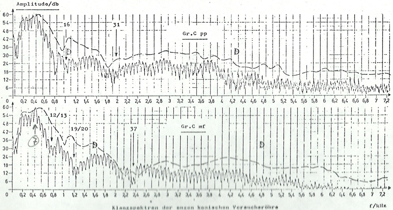
Klangspektren der engen konischen Versuchsröhre (Dulzianrohr)
