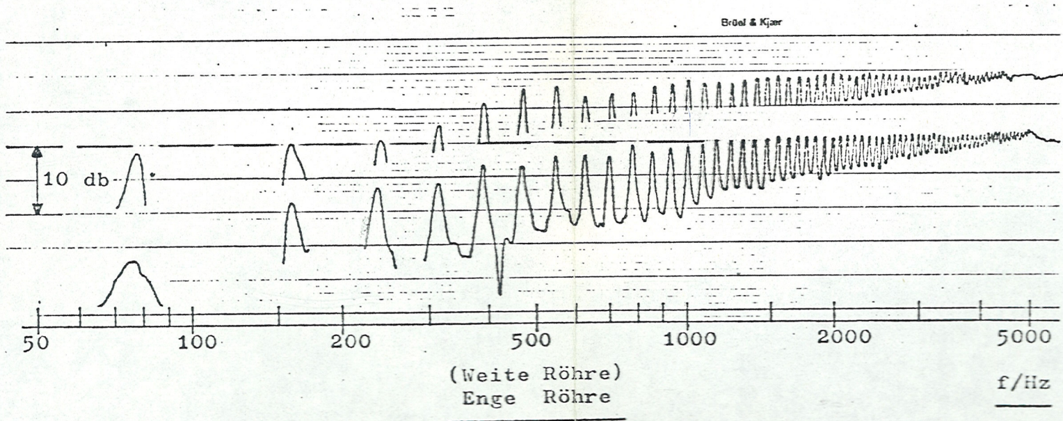
Eigenresonanzen der konischen Versuchsröhren
