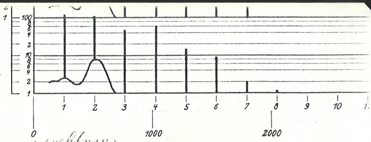
Abb. 18. Einfluß des Dämpfers.
