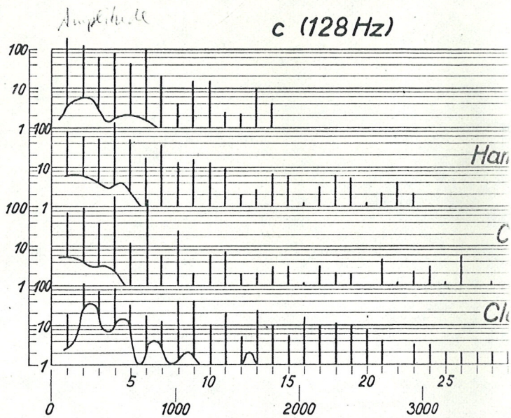
Abb. 19. Spektrum älterer klavierartiger Instrumente
