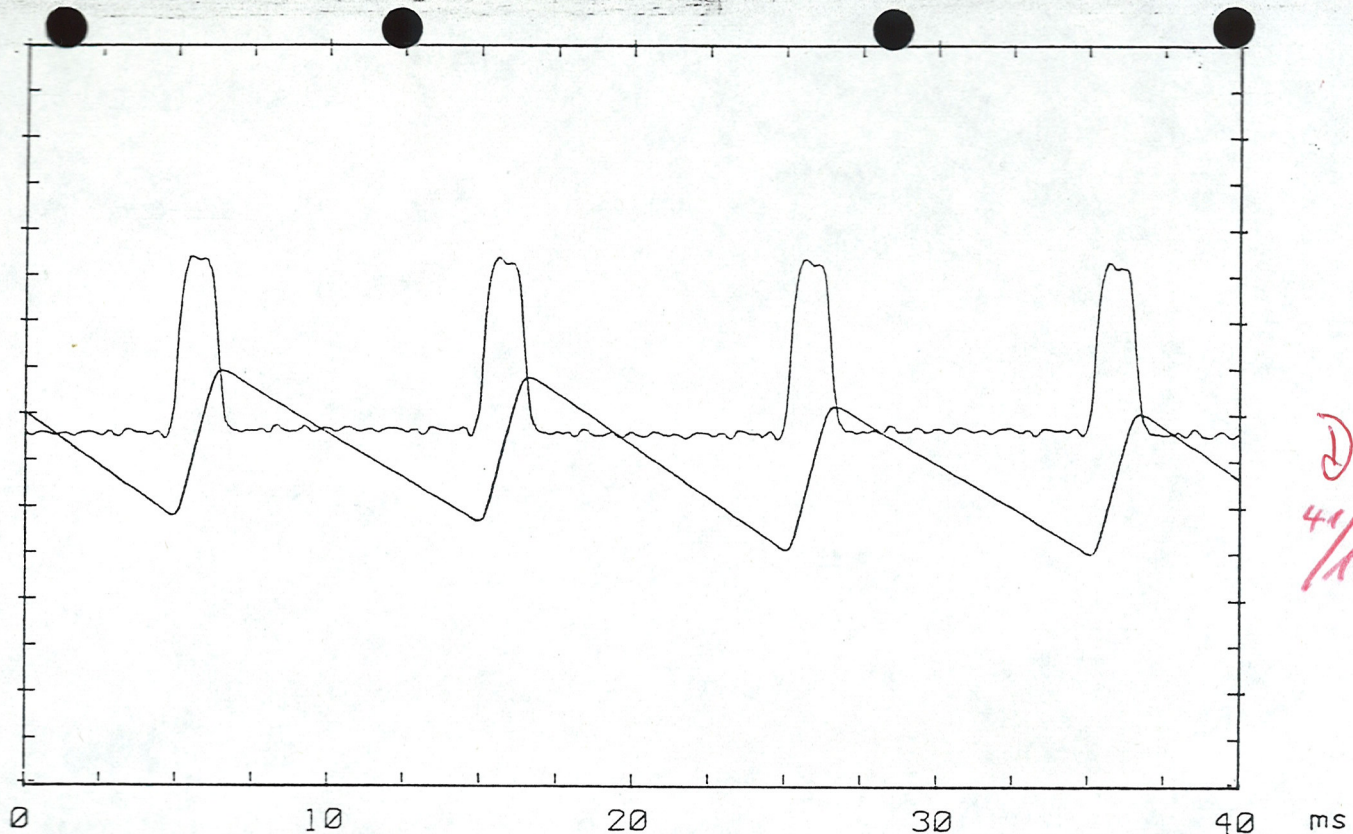
Schnelle (Impulsfolge) und durch Integration gewonnene Auslenkung (Sägezahn) an der Anstrichstelle (bei ca. 1/7 Saitenlänge) der leeren G-Saite ( f=99 Hz) des Kontrabasses für den Aufstrich.
