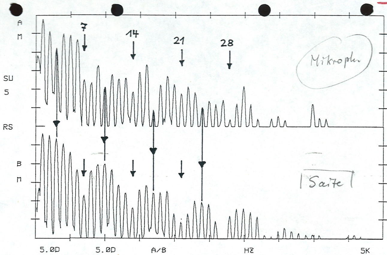
Bild 3: Spektrum des abgestrahlten Schalles (Mikrophonaufnahme, oben) und der Saitenschnelle an der Anstrichstelle (bei ca. 1/7 Saitenlänge, unten) von der G-Saite des Kontrabasses (99 Hz) Aufstrich.
