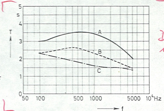
Abb. 76 (62) Musiksaal Stadt-Casino Basel, 1876. Nachhallzeiten. A leer, mit Holzbestuhlung (1936); B leer, mit teilweise gepolsterter Bestuhlung (1957); C mit Publikum.
