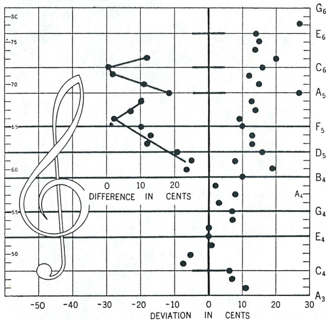
Abb. 1. Durchschnittliche Innenstimmung eines Alt-Saxophons in Es. Hersteller: C. G. Conn Limited Type und Nr.: 26 M Nr. 269 282 Mundstück: Conn Stealay Nr. 5 Stimmeneinrichtung auf Mittelstellung Spieler: L. E. Waddington Zimmertemperatur: 22 0 C Tage: 10.—23. September 1940 Testanzahl: 5
