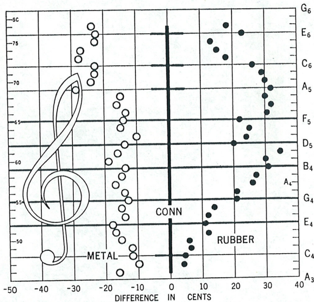
Abb. 2. Einfluß des Mundstückes auf die Innenstimmung eines Alt-Saxophons: Metallmundstück Otto Link Nr. 4* BB 37 und Gummimundstück Otto Link 9364 Nr. 4 im Vergleich mit dem Conn Steelay Nr. 5 Mundstück.
