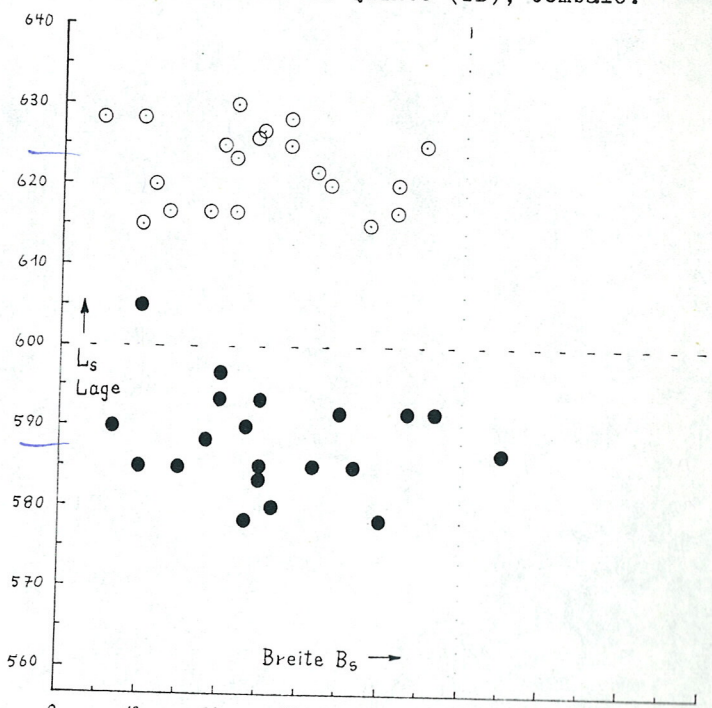
Abb. 24: Lage und Breite des Bereiches bevorzugter Intonationen bei übermäßiger Quarte (TH2) und verminderter Quinte (TI2); Geigen chor.
